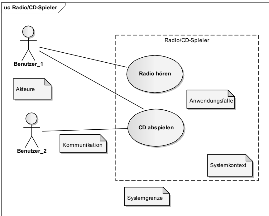
Abbildung 9-1: Anwendungsfalldiagramm
