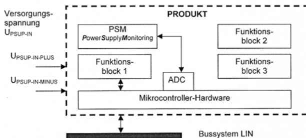
Abbildung 2-1: Blockschaltbild
