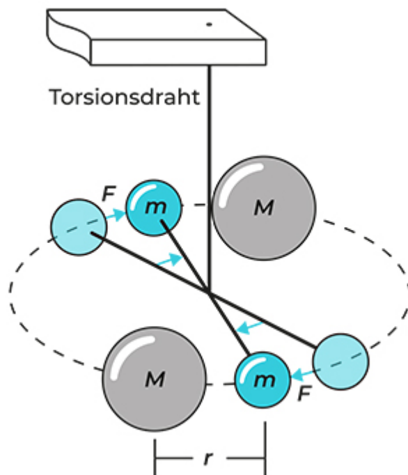
Abbildung 4.9: Henry Cavendishs Torsionswaage
