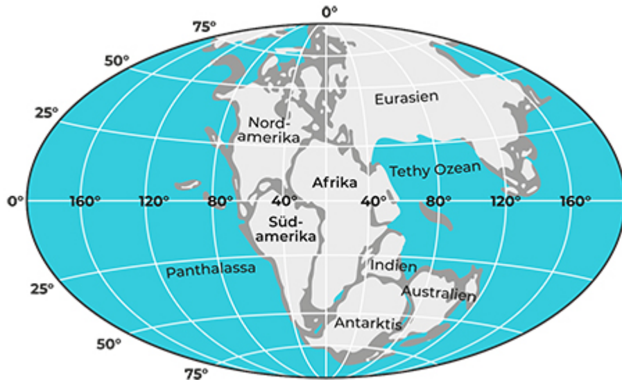
Abbildung 9.2: Der Urkontinent Pangaea, umschlossen vom Superozean Panthalassa
