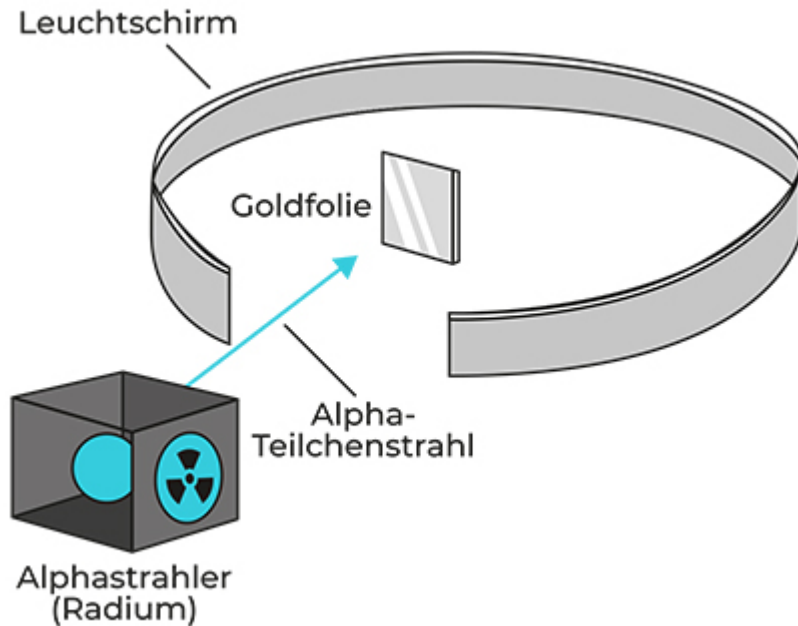
Abbildung 6.2: Aufbau des Goldfolien-Experiments
