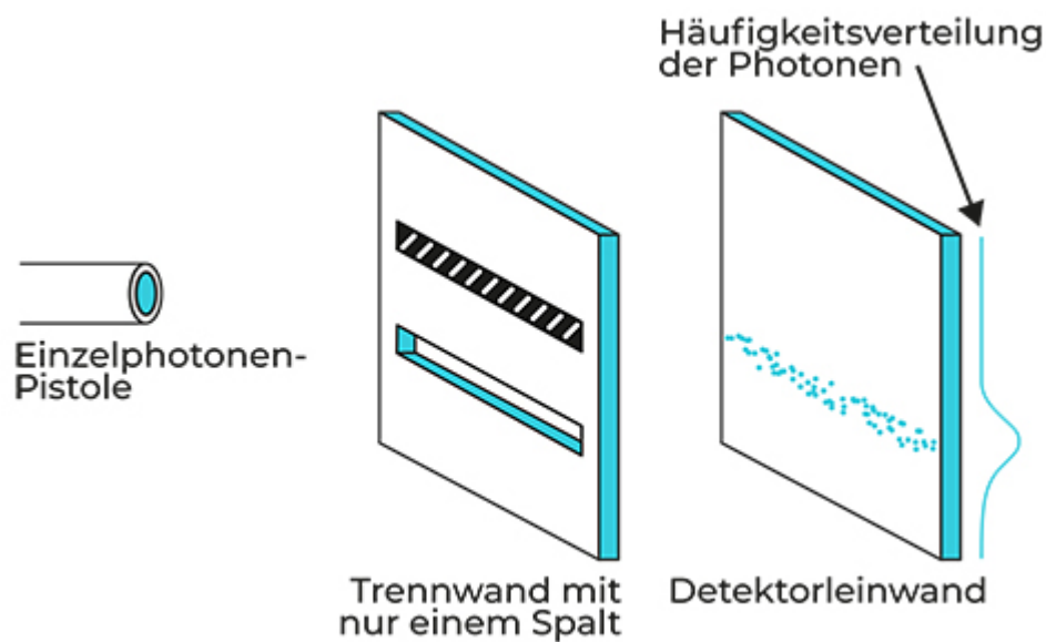
Abbildung 8.3: Photonen verhalten sich beim Einzelspaltexperiment wie Teilchen.
