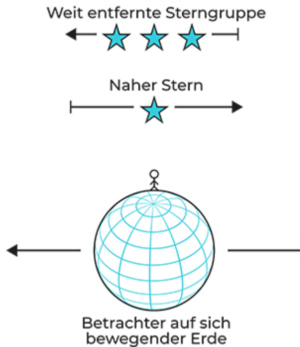
Abbildung 4.5: Stellare Parallaxe
