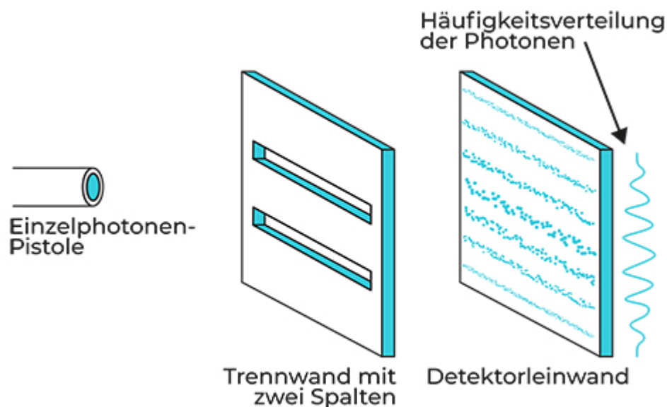
Abbildung 8.4: Photonen verhalten sich beim Doppelspaltexperiment wie Wellen.
