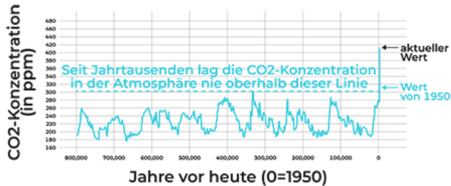
Abbildung 9.3: CO 2 -Konzentration in der Erdatmosphäre während der letzten 800000 Jahre
