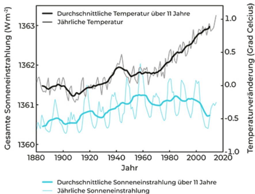
Abbildung 9.4: Schwankung der Sonnenaktivität (türkis) versus Anstieg der globalen Temperatur (schwarz)
