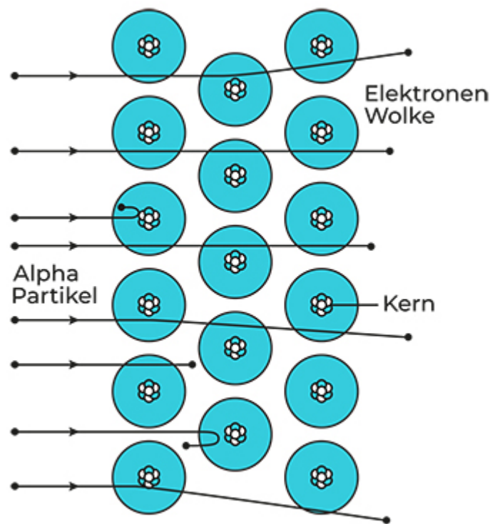
Abbildung 6.4: Ablenkung eines Alphateilchens im Goldfolien-Experiment
