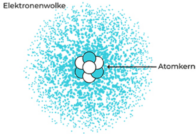
Abbildung 8.8: Atom nach Schrödinger: Die Elektronenwolke gibt die Wahrscheinlichkeit an, wo wir das Elektron finden können. Je dichter die Wolke, desto höher die Wahrscheinlichkeit.
