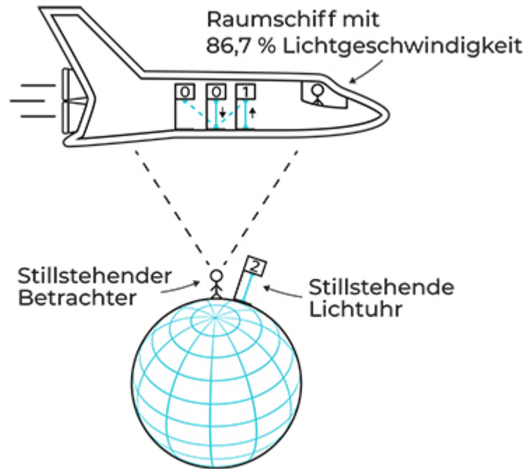
Abbildung 7.4: Die Lichtuhr bewegt sich
