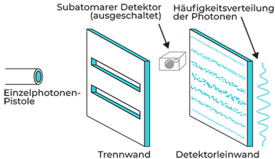
Abbildung 8.6: Das Doppelspaltexperiment mit deaktiviertem Detektor
