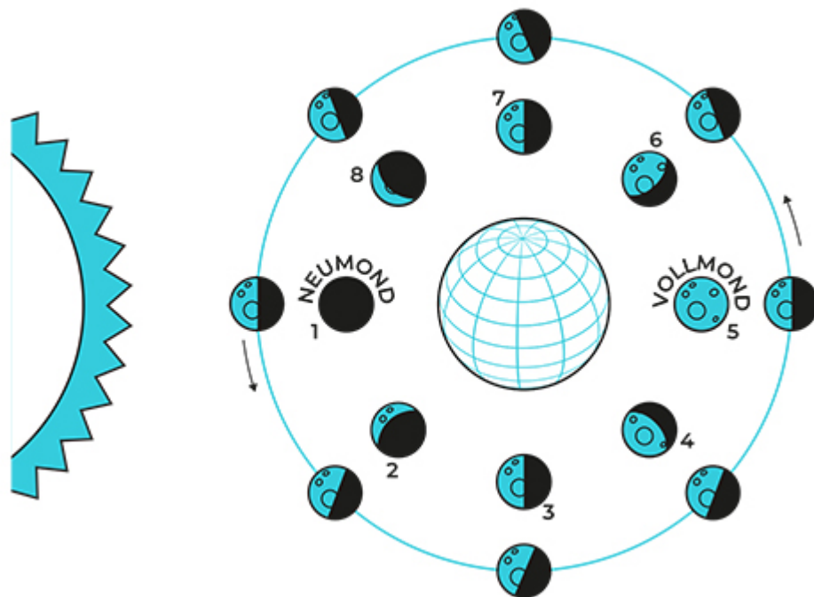
Abbildung 2.7: Mondphasen erklärt
