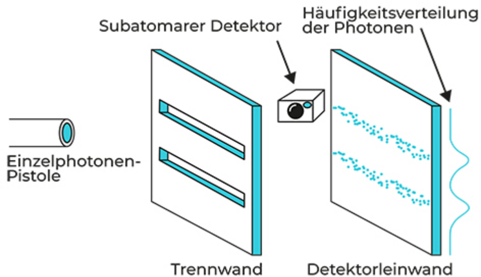
Abbildung 8.5: Doppelspaltexperiment mit Detektor
