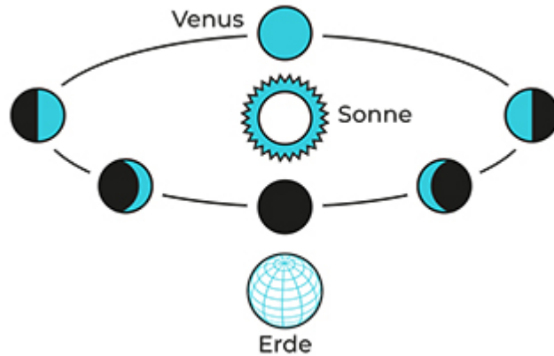
Abbildung 2.8: Venusphasen
