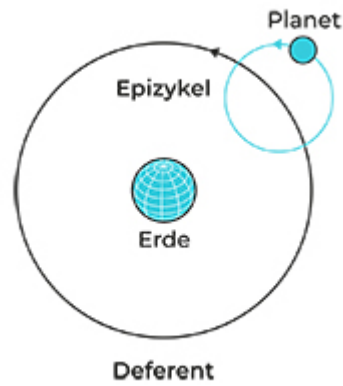
Abbildung 2.4: Epizykel
