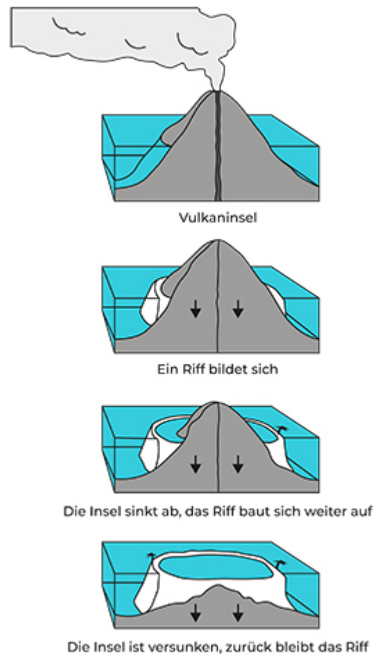
Abbildung 5.3: Entstehung eines Korallenatolls
