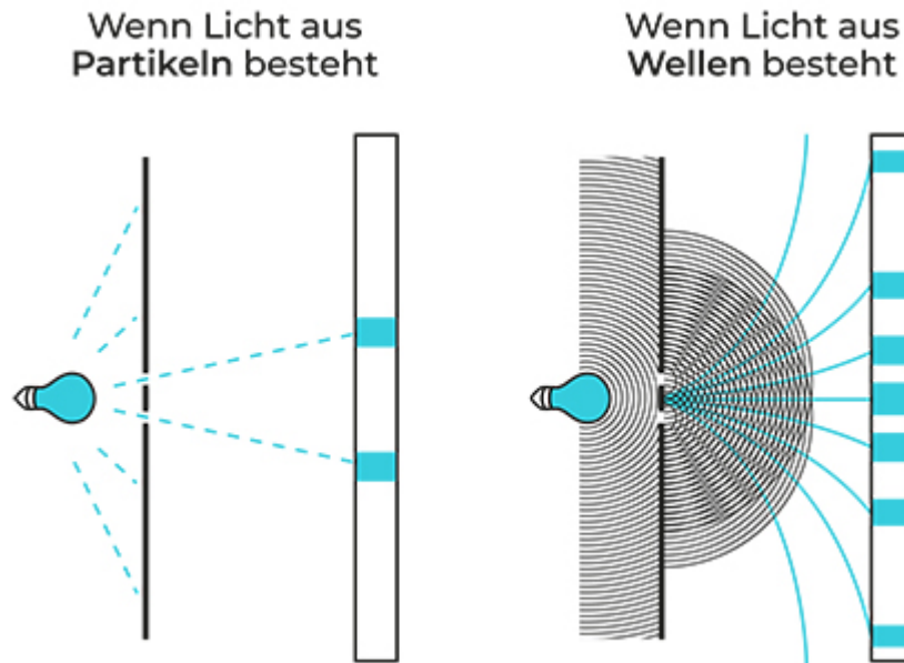
Abbildung 8.1: Zwei mögliche Ergebnisse des Doppelspaltexperiments: wenn Licht aus Teilchen besteht (links), wenn Licht aus Wellen besteht (rechts)
