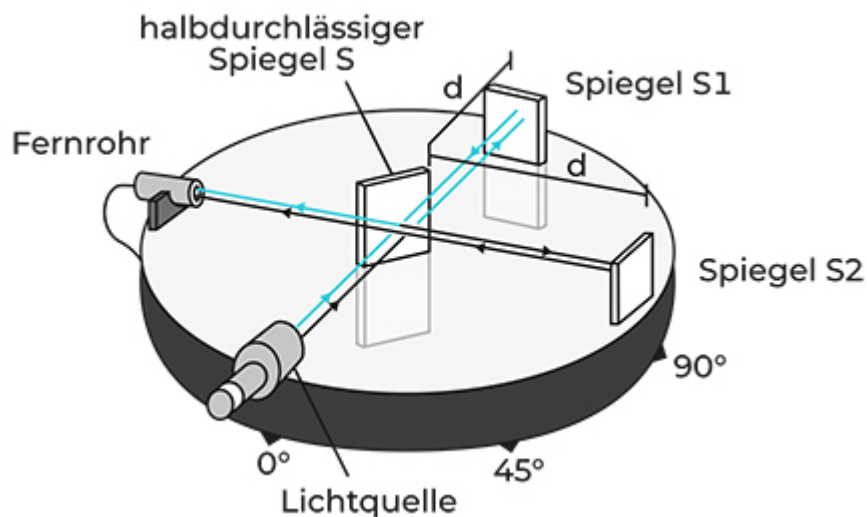
Abbildung 7.2: Das Michelson-Morley-Experiment
