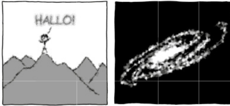
Atmosphärischer Dunst
